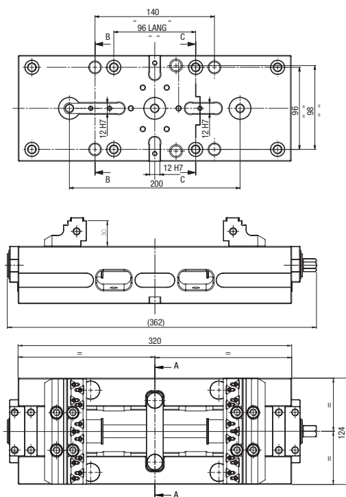
Autocentrante
