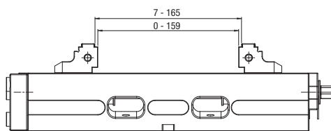
Fissa
