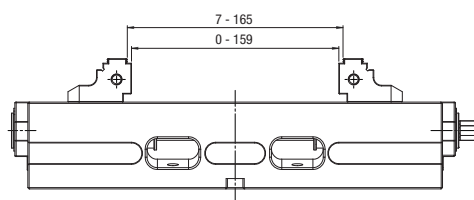
Doppio Bloccaggio
